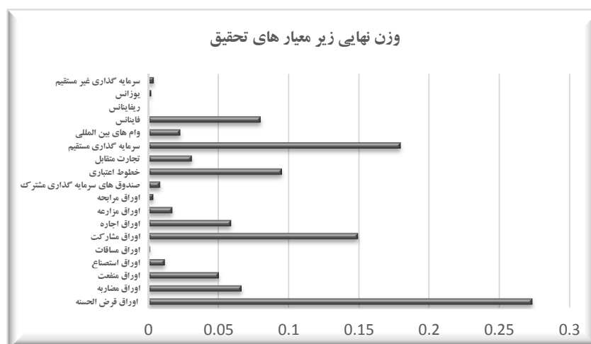
نمودار ۳. رتبه بندی نهایی زیر معیار های تحقیق
