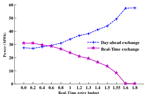
شکل ۷: انرژی مبادله شده با بازارهای روز پیشرو و زمان حقیقی در مقادیر مختلف بودجه قیمت بازار زمان حقیقی
