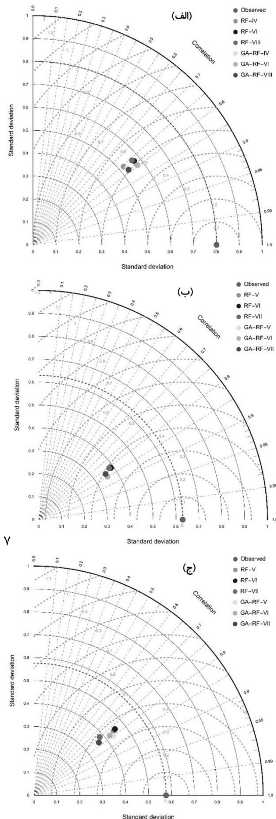
شکل ۷- دیاگرام تیلور تابش خورشیدی مشاهداتی و پیش‌بینی شده با استفاده از سه سناریو برتر هر ایستگاه: الف) گرمی، ب) مشگین شهر، و ج) نیر
