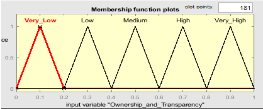
شکل (۳) – تابع عضویت متغیر ورودی مالکیت و شفافیت منبع: یافته های پژوهشگر
