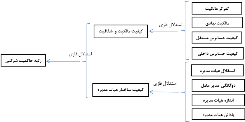
شکل (۱) - مدل تحقیق منبع: یافته‌های پژوهشگر
