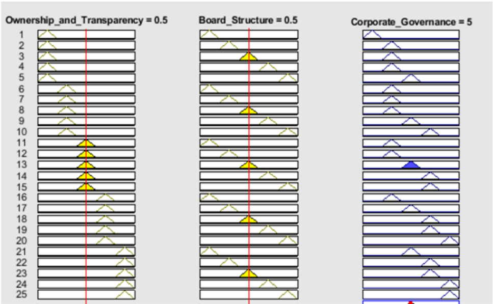
شکل (۱۳) - نمایش پایگاه قواعد فازی برای به هم پیوستن شاخص مالکیت و شفافیت و شاخص ساختار هیات مدیره منبع: یافته‌های پژوهشگر
