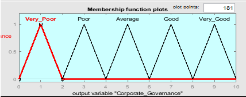
شکل (۵) – تابع عضویت متغیر خروجی کیفیت حاکمیت شرکتی منبع: یافته های پژوهشگر
