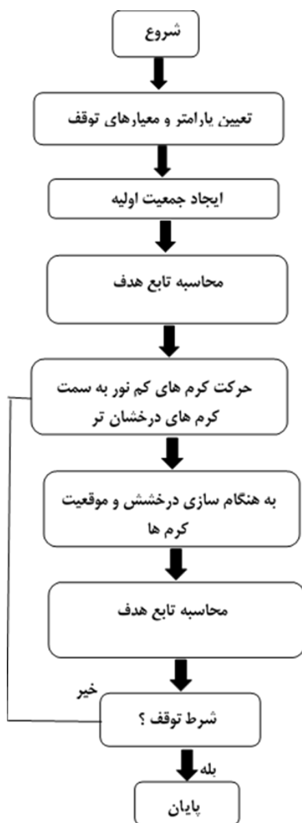
شکل ۴. فلوجارت الگوریتم کرم شب‌تاب
