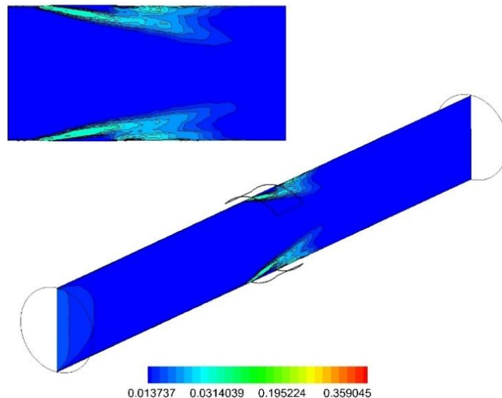
شکل ۱۳- خطوط هم‌تراز انرژی جنبشی آشفته‌گی به ازای شدت میدان مغناطیسی ۰/۰۳
