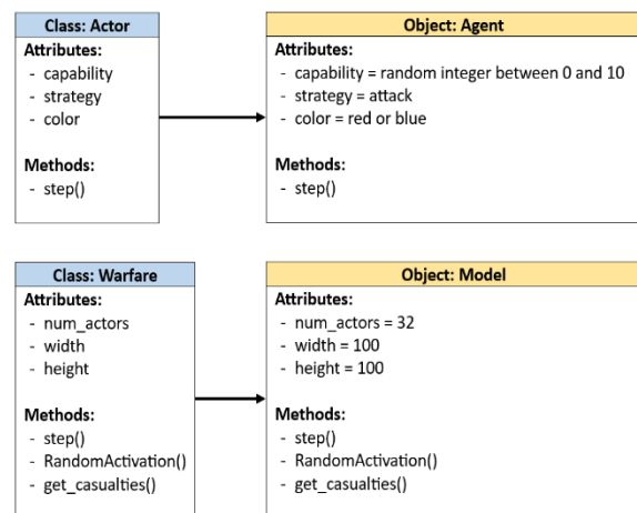
شکل (۲): طرح کلاس پیشنهادی برای الگوسازی بازی جنگ متعارف
