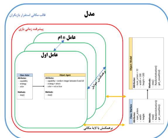
شکل (۳): ساختار مفهومی چارچوب الگوسازی بازی جنگ متعارف
