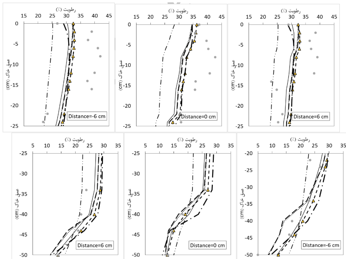
شکل ۳- تغییرات رطوبت اندازه‌گیری و شبیه‌سازی شده در زمان ۲۴ ساعت پس از آبیاری قطره‌ای سطحی برای ۵ مدل موجود در نرم‌افزار HYDRUS-2D و مدل BMA.
