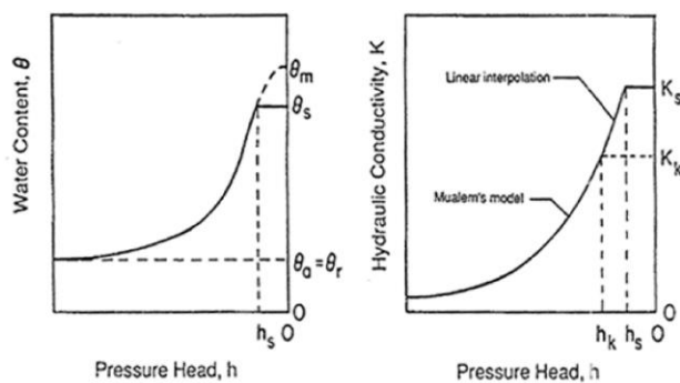
شکل ۱- توابع نگهداشت آب خاک و هدایت هیدرولیکی ارائه شده در
