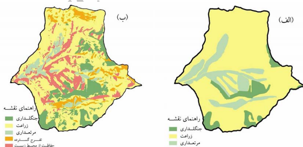
شکل ۶. نقشه کاربری فعلی (الف) و نقشه توان اکولوژیک (کاربری آتی) (ب) حوضه کچیک
