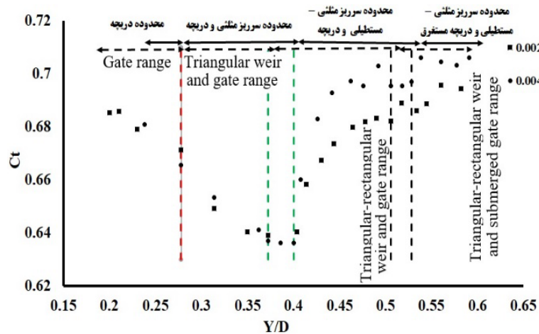
Fig.12 Checking the flow coefficient in the dimensionless opening 0.09 in two slopes 0.002 and 0.004 شکل ۱۲ بررسی ضریب دبی در بازشدگی بی‌بعد ۰/۰۹ در دو شیب ۰/۰۰۲ و ۰/۰۰۴
