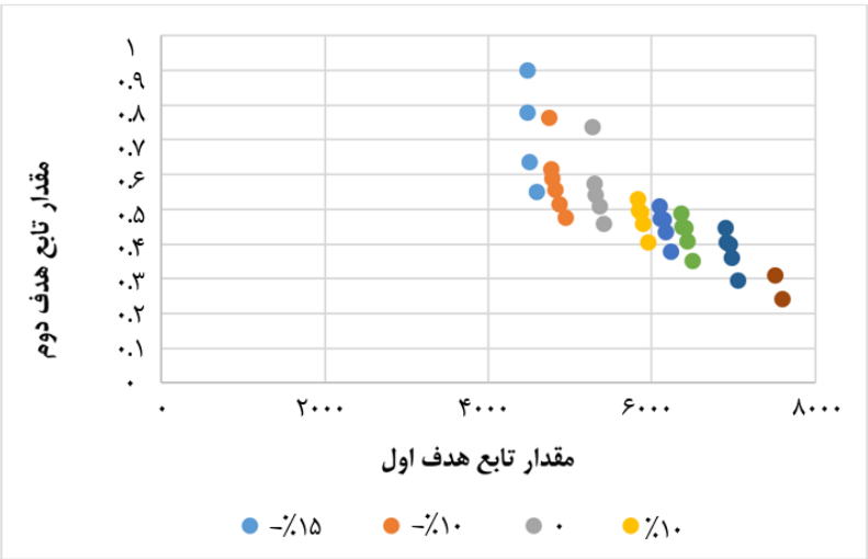
شکل ۶. تغییرات توابع هدف به‌ازای درصدهای تغییر در سرعت پیشرانه پهباد
