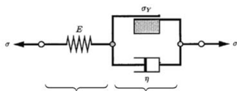
شکل ۳- ساختار ریاضی یک ماده ویسکوپلاستیک [۲۵].
