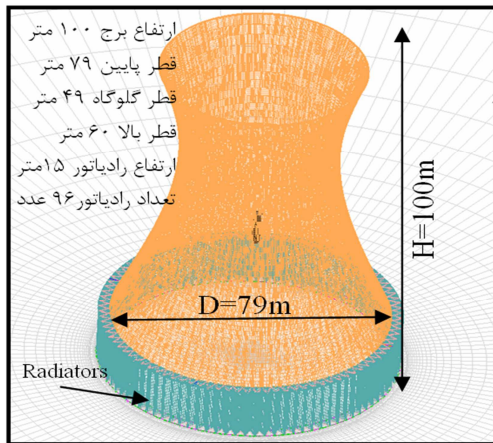
شکل ۱- طرحواره برج هالر مورد مطالعه (نیروگاه چرخه ترکیبی فارس)
