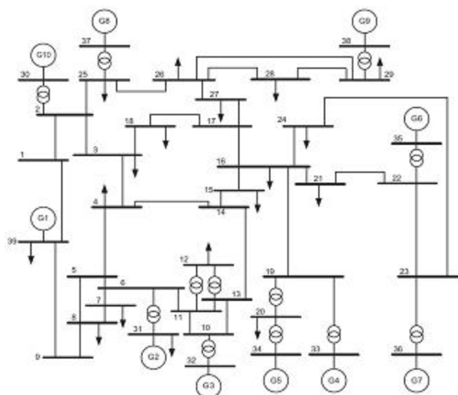
شکل (۴): دیاگرام تک خطی سیستم ۳۹ باسهای جدید انگلیس
