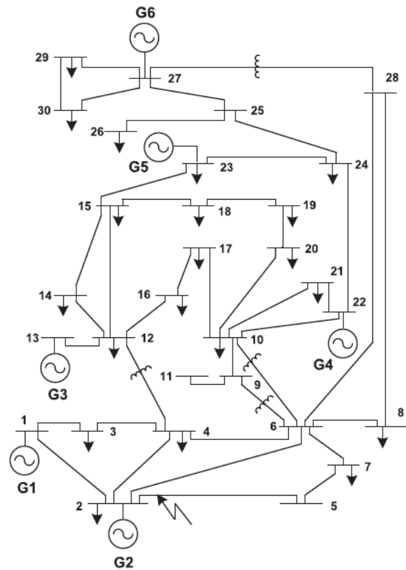
شکل (۶) شبکه تست سی باسه IEEE
