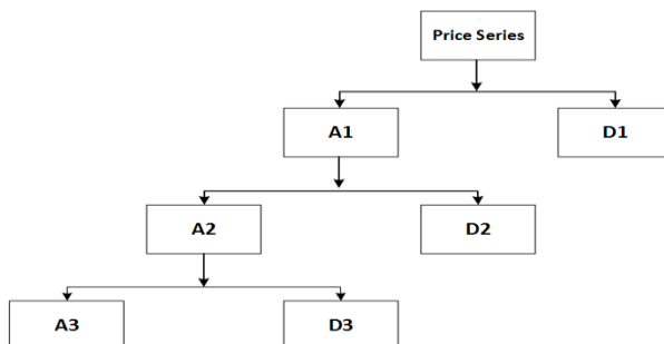
شکل ۱- درخت تجزیه شده با تبدیل موجک تا سطح ۳
