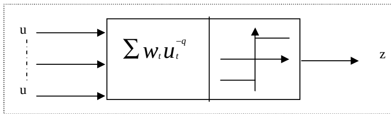
نمودار 1: نرون مصنوعی با تابع آستانه
