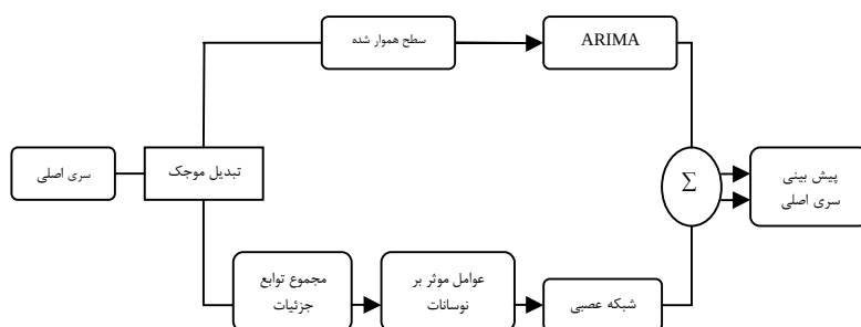
نمودار 3: ساختار مدل ترکیبی موجک
