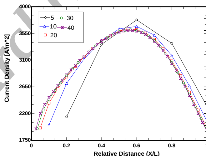
شکل ۶- بررسی تاثیر تعداد المان در امتداد کانال‌ها بر روی توزیع چگالی جریان
