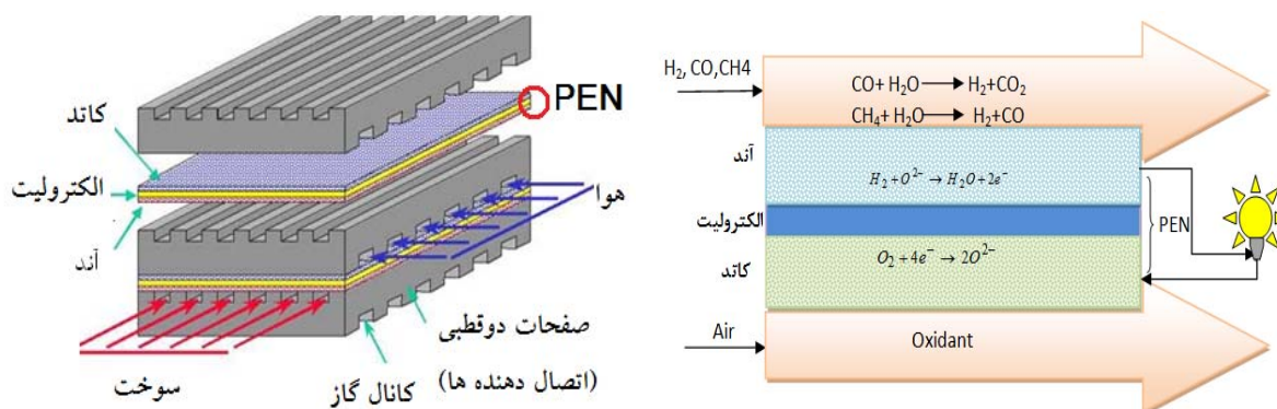
شکل ۲- پیل سوختی اکسید جامد با ساختار صفحه‌ای
