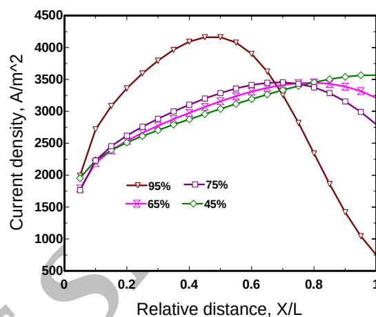
شکل ۷- بررسی تاثیر فاکتور مصرف سوخت بر روی چگالی جریان خروجی
