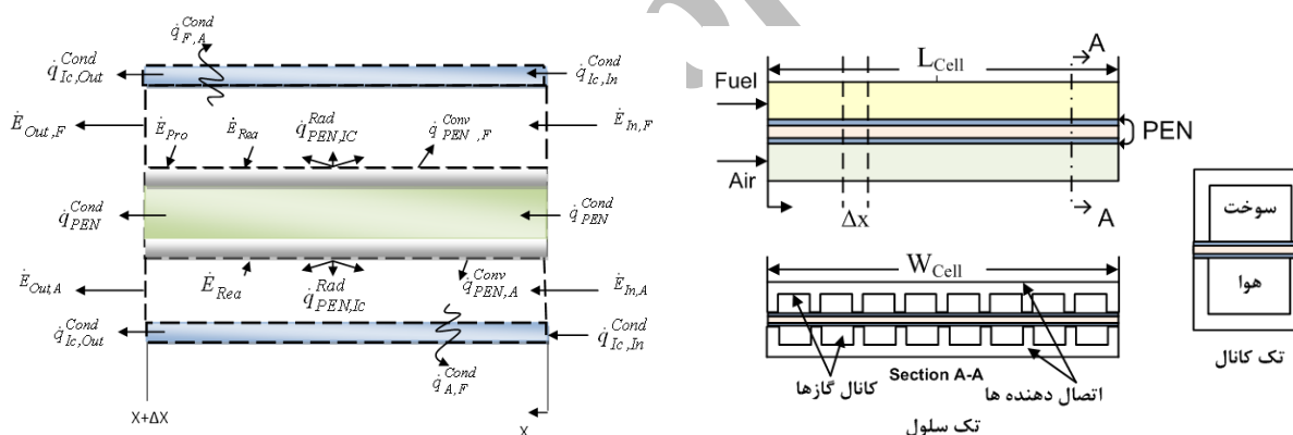
شکل ۴- بالانس انرژی برای یک المان در حجم کنترل با در نظر گرفتن ۵ لایه دهانه
