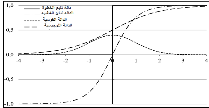
الشكل 04: أنواع دوال التنشيط
