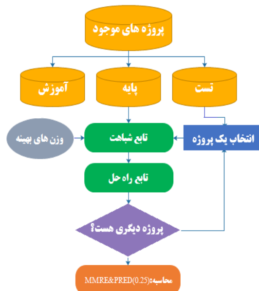
شکل ۷: فلوچارت مربوط به گام آزمون مدل پیشنهادی
