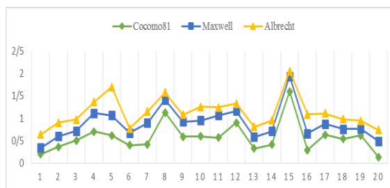
نمودار ۹: نتایج MdmRE بدست آمده بر روی سه مجموعه داده توسط مدل CBR+PSO
