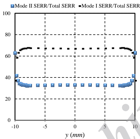
شکل ۱۲- منحنی توزیع نسبت موده‌های چقرمگی شکست به مقدار کلی آن در راستای عرض نمونه با h_1 / h_2 = 0.33
