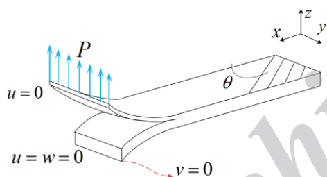
شکل ۶- شرایط بارگذاری و مرزی نمونه مدل‌سازی شده
