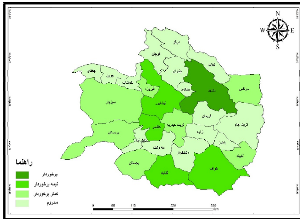
شکل ۱: سطح بندی نهایی مناطق استان از لحاظ برخورداری از شاخص‌های تلفیقی توسعه
