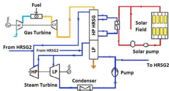
شکل (۱): طرح‌واره چرخه ترکیبی خورشیدی مورد مطالعه [۱۵]
