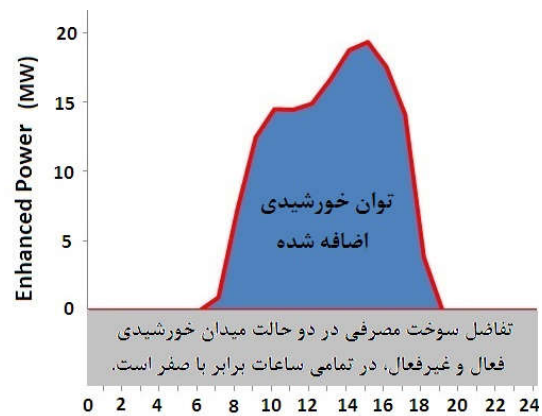
شکل (۳): توان خورشیدی اضافه شده به چرخه در ساعات مختلف روز طراحی بر حسب مگاوات
