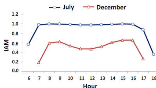
شکل (۱۰): ضریب تصحیح زاویه تابش در ساعات مختلف روز میانگین دو ماه جولای و دسامبر
