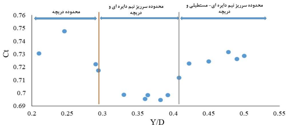
شکل ۰۵. ضریب دبی در بازشدگی ۷/۵ سانتی متری دریچه با دبی‌های متفاوت
