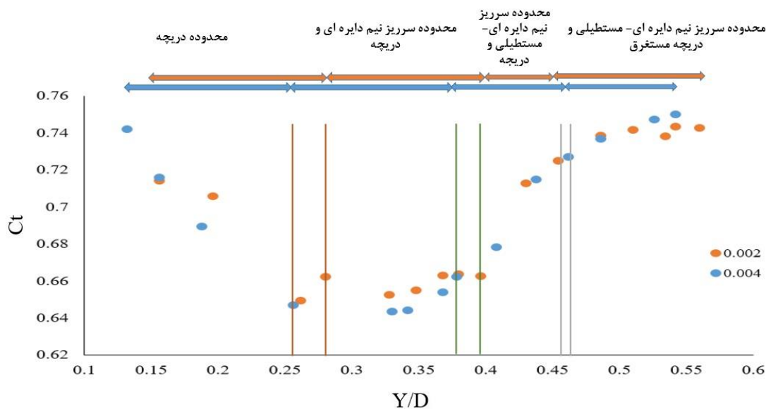
شکل ۱۴. بررسی ضریب دبی در بازشدگی ۴/۵ سانتی‌متر در دو شیب ۰/۰۰۲ و ۰/۰۰۴
