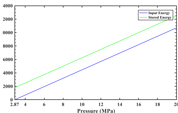
شکل 16 افزایش انرژی ورودی و ذخیره‌شده مخزن با افزایش فشار در طول فرآیند شارژ
