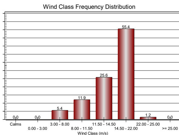
شکل 7 کلاس‌های باد در منطقه خواف در بازه زمانی هفتم تا سیزدهم جولای 2008
