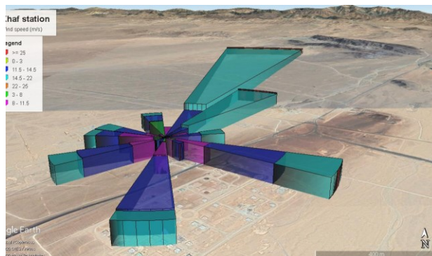
شکل 6 گلباد در تصویر هوایی ایستگاه خواف در بازه زمانی هفتم تا سیزدهم جولای 2008
