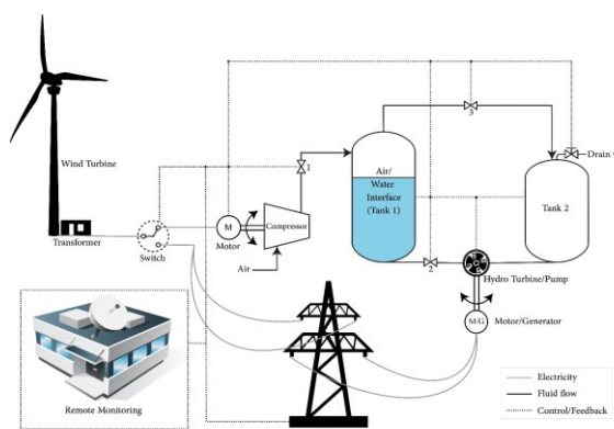
شکل 1 طرح‌واره سیستم ارائه‌شده متصل به نیروگاه بادی و شبکه برق
