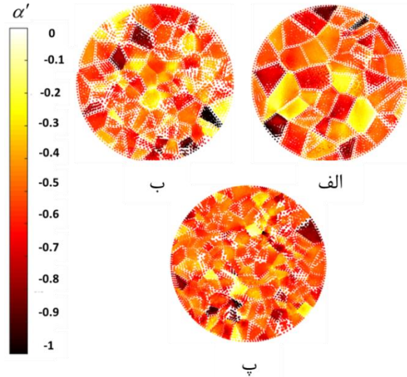
شکل (۵): مقدار نسبت کرنش عرضی ( \varepsilon_{YY} ) به کرنش طولی ( \varepsilon_{XX} ) پس از تغییر شکل نمونه‌های متشکل از الف (۵۰ دانه، ب) ۱۰۰ دانه و پ) ۲۰۰ دانه پس از ۵۰٪ کاهش ارتفاع در آزمون فشار
