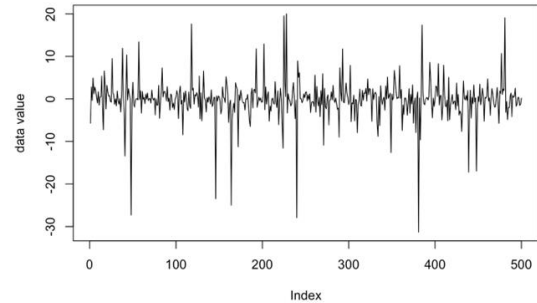
شکل ۳. داده‌های شبیه‌سازی شده با توزیع تی استیودنت (درجه آزادی = ۵)
