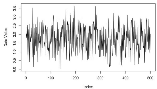
شکل ۵. داده‌های شبیه‌سازی شده با توزیع ویبول (شکل ۵ و مقیاس ۲)
