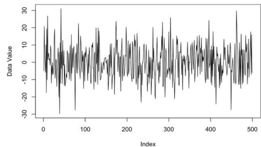
شکل ۴. داده‌های شبیه‌سازی شده با توزیع نرمال (میانگین صفر و انحراف معیار = ۴)
