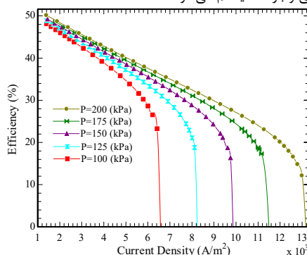
شکل ۱۳- تغییرات بازده سیستم در فشارهای مختلف با چگالی
