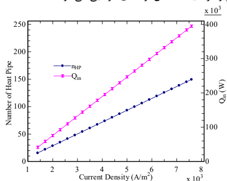
شکل ۵- اثر تغییرات چگالی جریان بر گرمای لازم و تعداد لوله‌های گرمایی مورد نیاز
