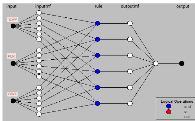
شکل ۶- مدل نروفازی به دست آمده برای پیرومتر مرکزی دشت
