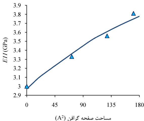
شکل ۷ نمودار سفتی در راستای ۱ بر حسب مساحت صفحه گرافن
