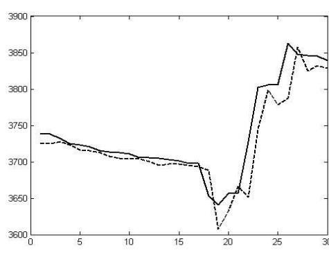
شکل (۴): پیش بینی قیمت سهام با استفاده از یک شبکه عصبی MLP ساده و مدل ترکیبی شرکت سیمان شرق
