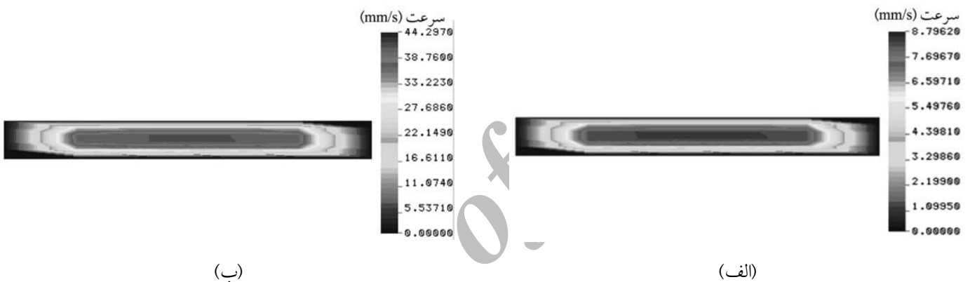
شکل ۸- نیم رخ سرعت در خروجی حدیده برای نمونه PE-0200 در سرعت های مختلف پیچ: (الف) 20 rpm و (ب) 100 rpm.
