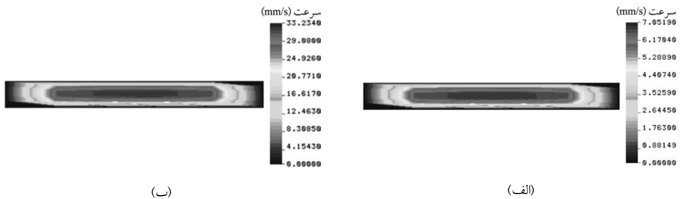
شکل ۹- نیم رخ سرعت در خروجی حدیده برای نمونه PE-EX3 در سرعت های مختلف پیچ: (الف) 20 rpm و (ب) 100 rpm.
