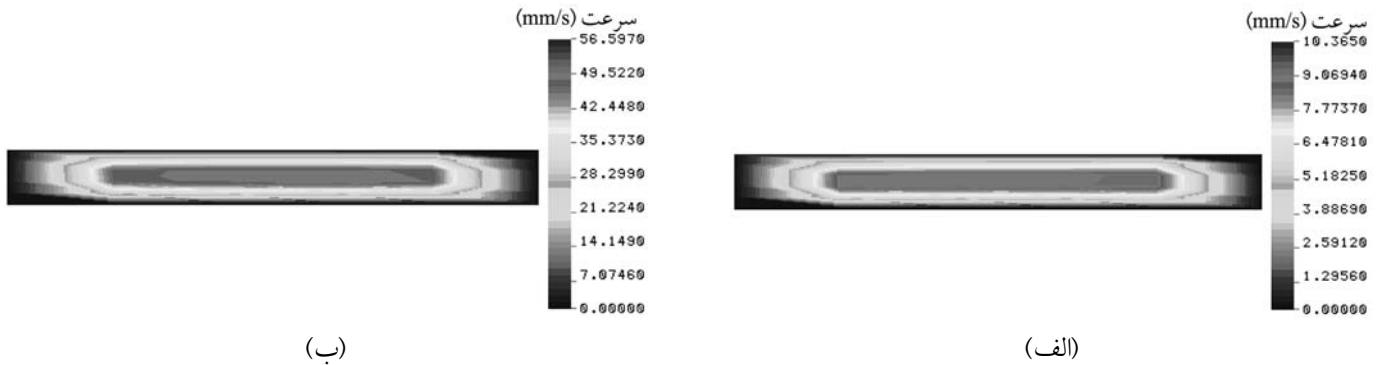
شکل ۷- نیم رخ سرعت در خروجی حدیده برای نمونه PE-5218 در سرعت های مختلف پیچ: (الف) 20 rpm و (ب) 100 rpm.
