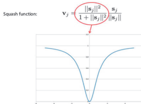
شکل ۷. شکل تابع Squash منبع: Candemir et al., 2014
