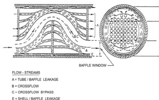
شکل ۳. جریان‌های مؤثر سمت پوسته طبق مدل تینکر [۴]
