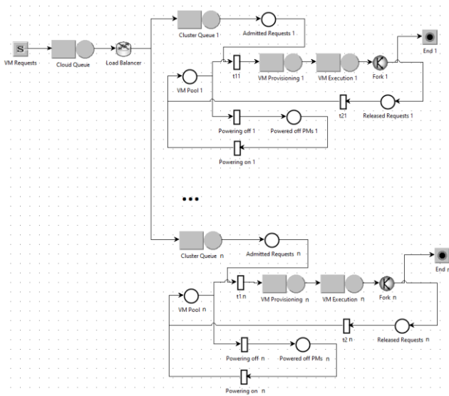
شکل ۳: مدل تحلیلی یکنوای ارائه شده برای مرکز داده ابری
