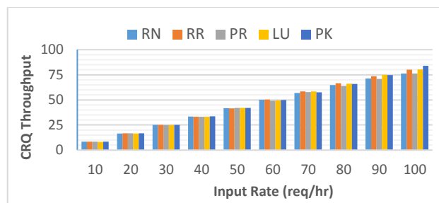
شکل ۱۰: توان عملیاتی صف‌های CRQ کلاسترها
