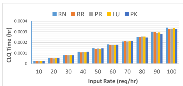
شکل ۱۱: زمان انتظار درخواست‌ها در صف CLQ ابر
