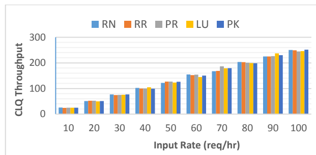
شکل ۹: توان عملیاتی صف CLQ ابر
