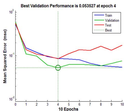
Levenberg -Marquardt
