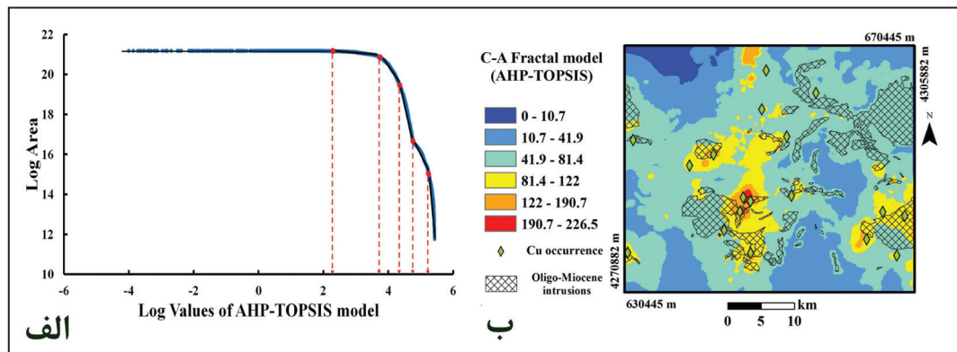
شکل ۶- الف) نمودار تمام لگاریتمی عیار- مساحت؛ ب) نقشه کلاسه بندی شده با استفاده از روش فرکتال عیار- مساحت در مدل سازی پتانسیل کانی زایی مس پورفیری در بخش مرکزی ورزقان با استفاده از روش AHP-TOPSIS.
