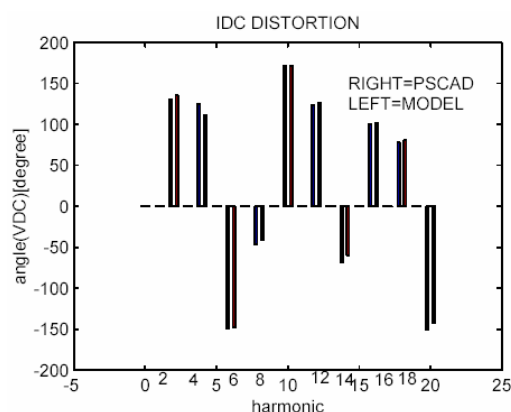
شکل ۵-ب- فاز هارمونیکهای ولتاژ DC در حالت اعوجاج جریان DC
