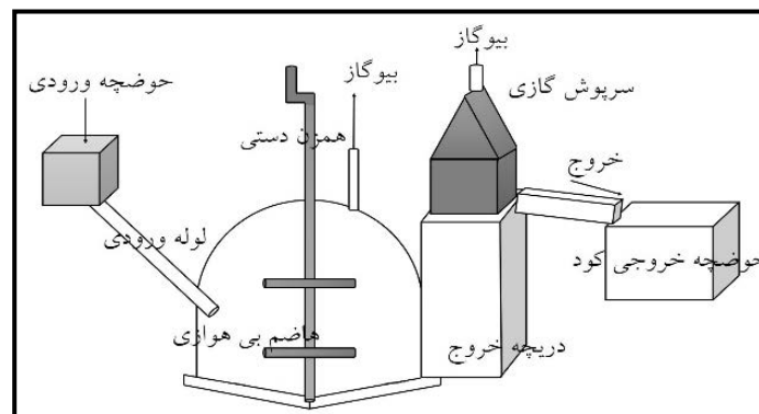
شکل ۴- راکتور بی‌هوازی ترکیبی چینی و هندی
