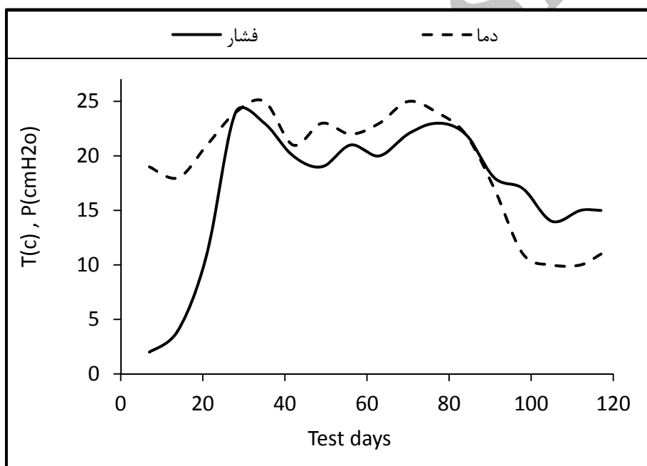
شکل ۱۶- دما و فشار اندازه گیری شده تجربی رآکتور
