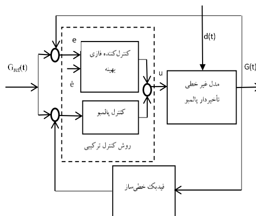
شکل ۱: دیاگرام بلوکی کنترل ترکیبی فیدبک خطی ساز- هوشمند
