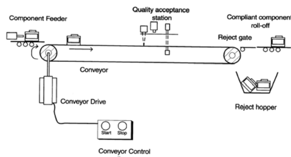
شکل (۵): شماتیک سیستم نورد تست قطعات [۲]
