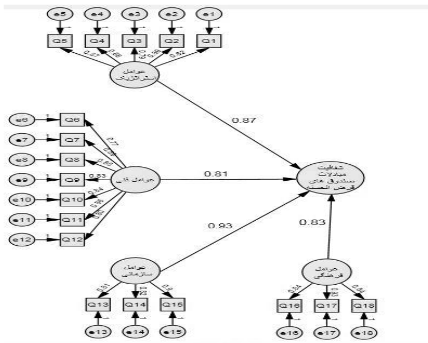
شکل ۸. مدل معادلات ساختاری (در حالت استاندارد)
